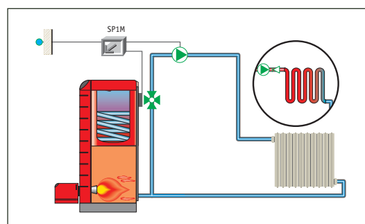
Schéma d'installation d'un radiateur pour régulation ECOCONTROL/SP 1 M
